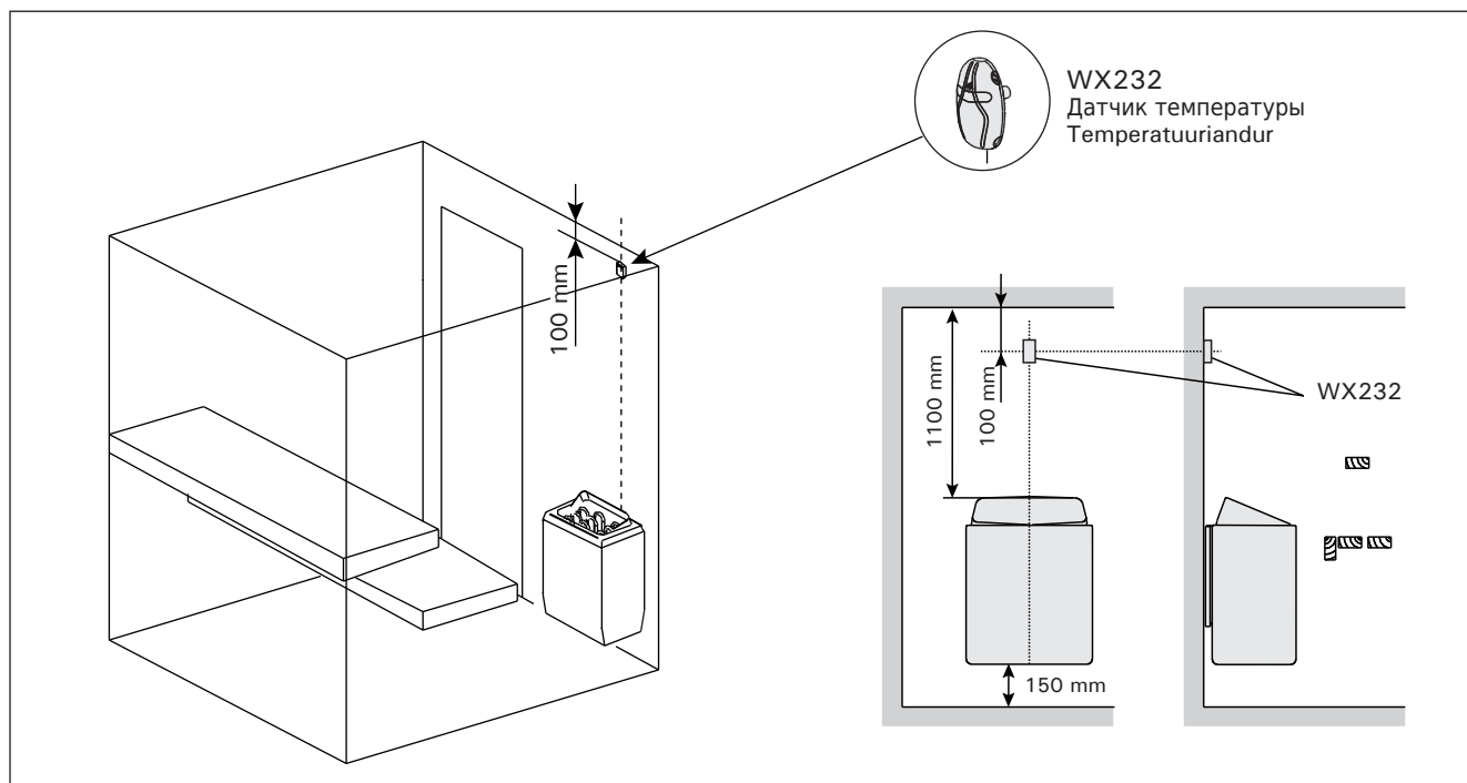
Рисунок 7. Расположение датчиков температуры относительно настенных нагревателей
